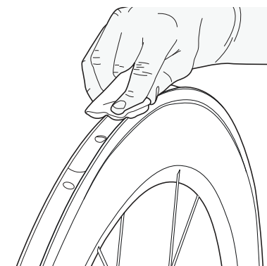
Figure 21. Essuyez la zone poncée de la jante avec un chiffon propre et une petite quantité d'acétone et préparez-la pour la colle.
